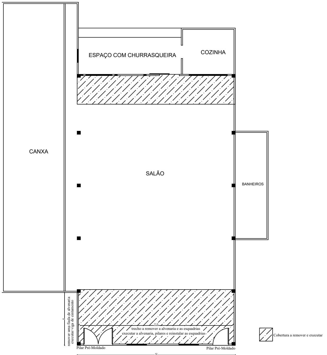
PLANTA BAIXA ESCALA 1:75
